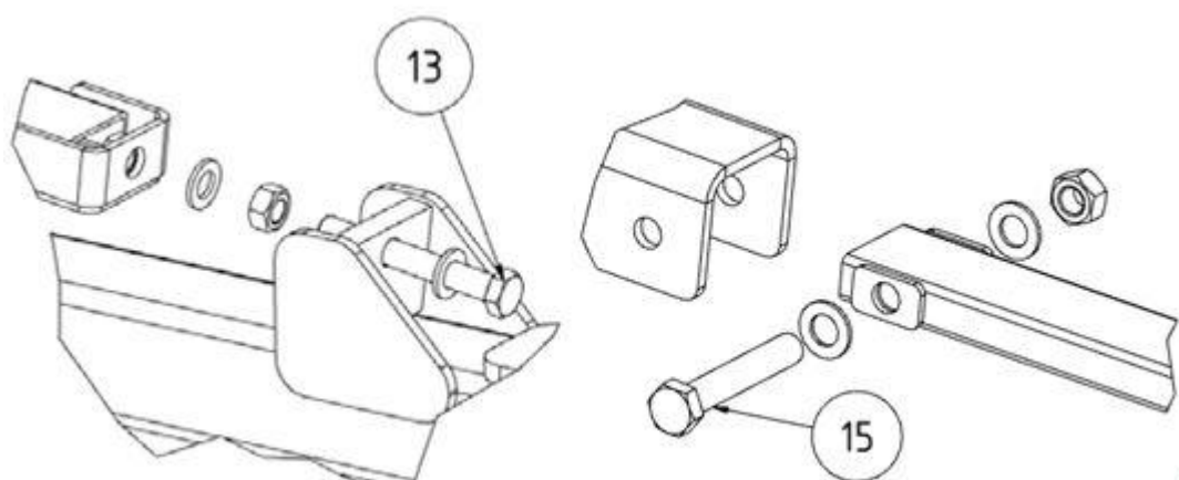
Obr. 8: Prodlužovací rameno
