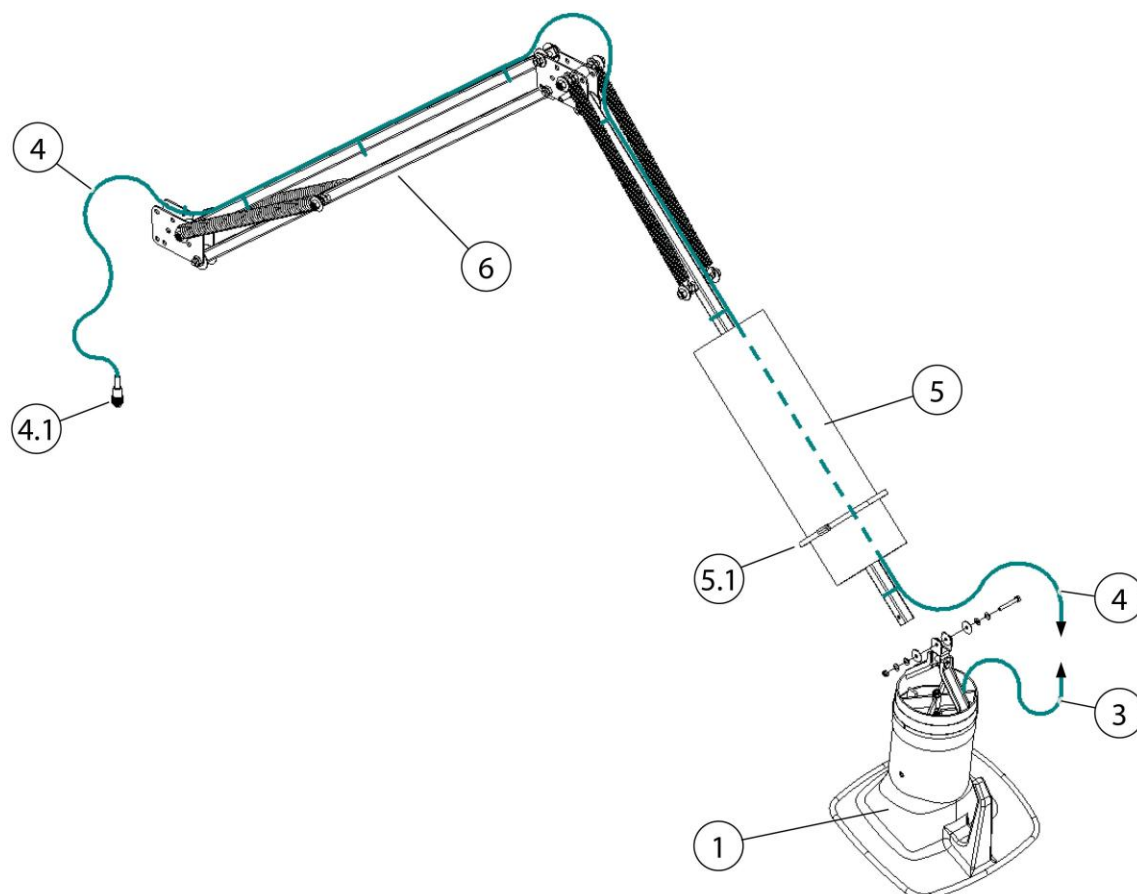
Obr. 18: Pokládka kabelů – odsávací rameno 2-4 m
