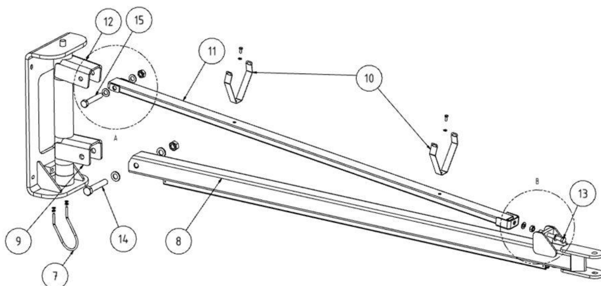
Obr. 7: Prodlužovací rameno část 1
