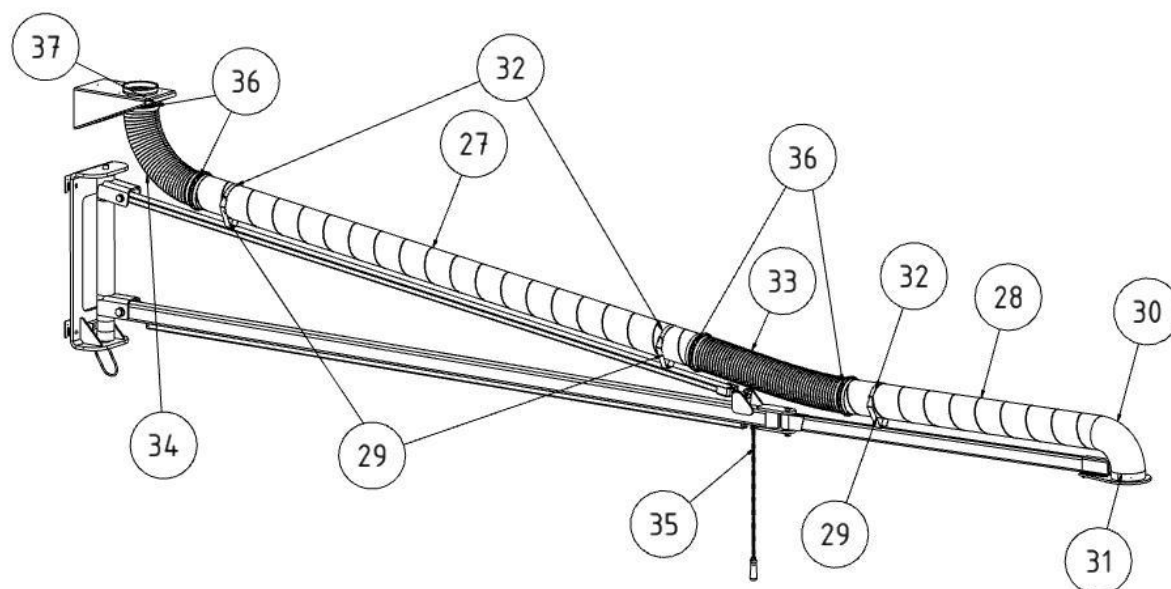
Obr. 14: Montáž spiro trubky
