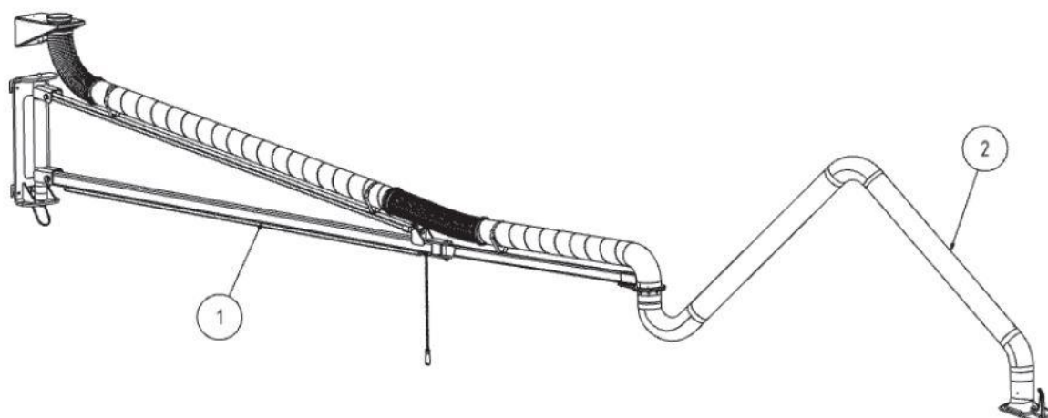
Obr. 3: Prodlužovací rameno s odsávacím ramenem
