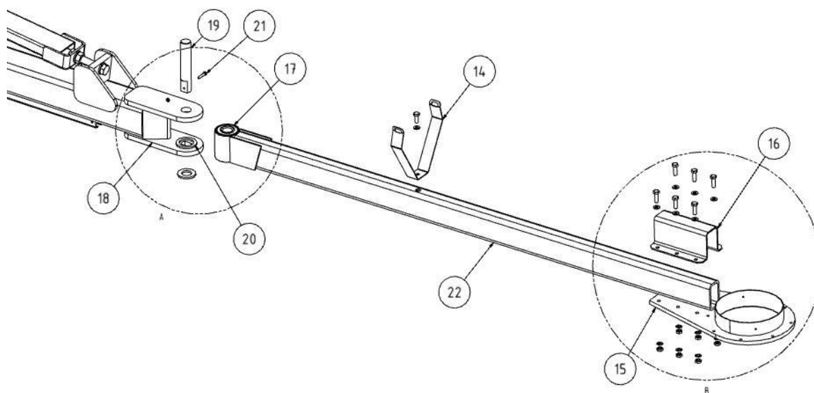
Obr. 9: Prodlužovací rameno část 2
